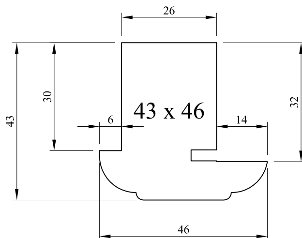
° Profil au dessus du pivot
