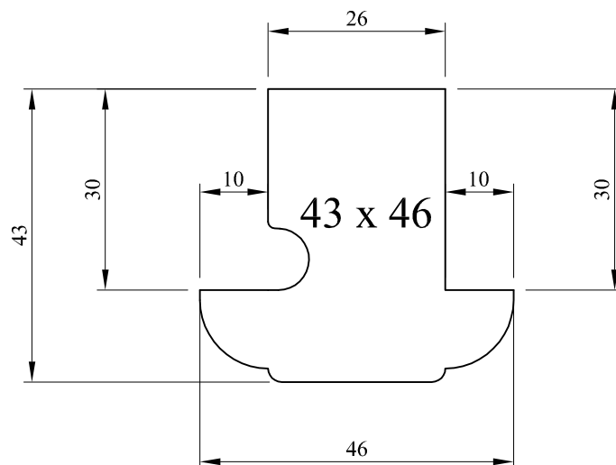
° Profil au dessous du pivot
