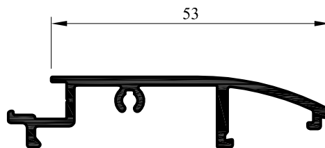
Réf 3010202 (remplissage de 24mm)
