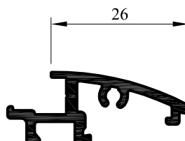
Réf 3010198 (remplissage de 24mm)
