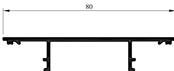
Réf 3010188 (Parclose pour traverse ou montant intermédiaire)
