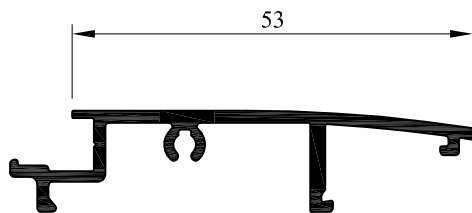
Réf 3010179 (remplissage de 28mm)
